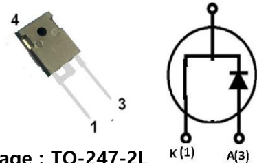
Package : TO-247-2L
