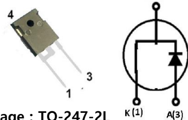
Package : TO-247-2L
